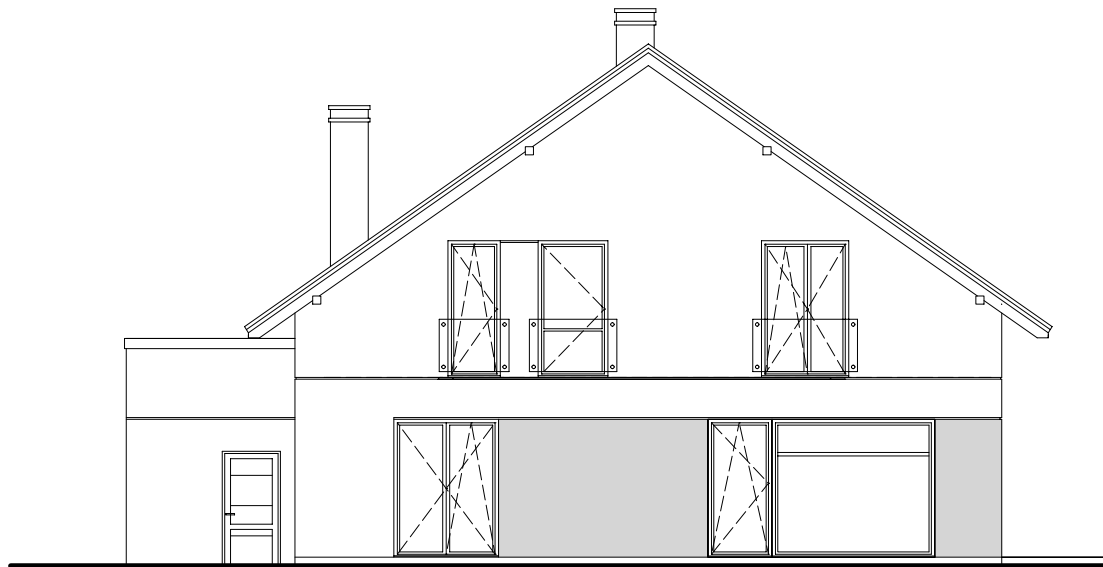
ELEWACJA OGRODOWA
